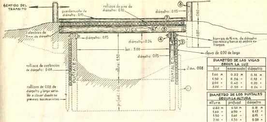
Figura 1 — Corte longitudinal — Escala: 1: 25
